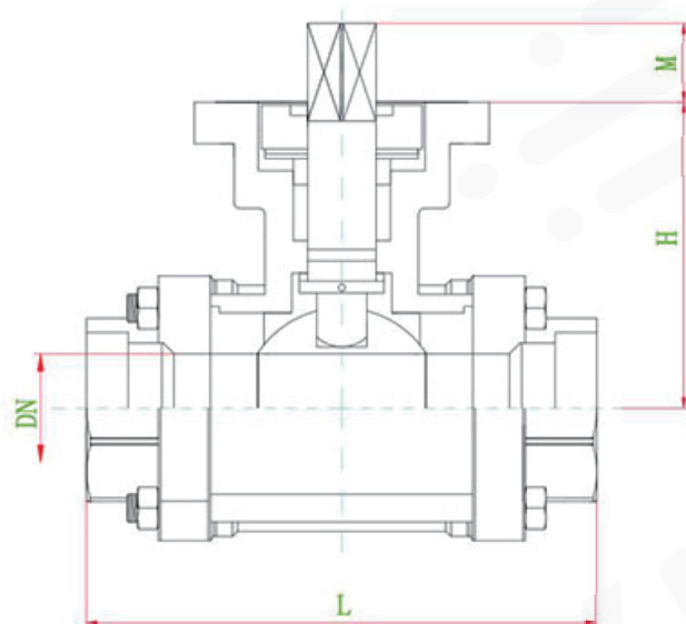
三片式螺纹
