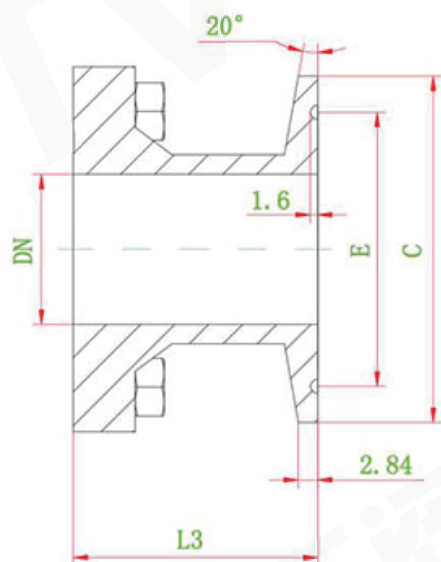
三片式卡箍
